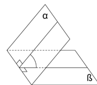
მახვილი კუთხე 0^\circ < \varphi < 90^\circ
