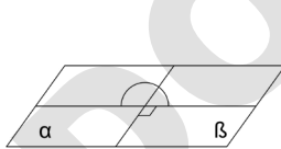
გაშლილი კუთხე \varphi = 180^\circ
