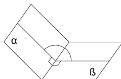
ბლაგვი კუთხე 90^\circ < \varphi < 180^\circ
